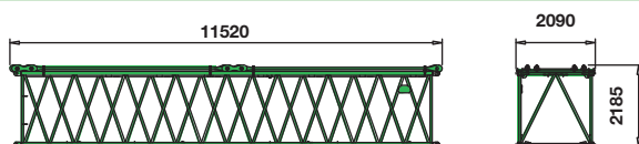
Auslegerzwischenstück 11,2 m Typ SH 2008 (mit SH/SHWS Abspannung) Boom insert 11.2 m type SH 2008 (with SH/SHWS pendants)
